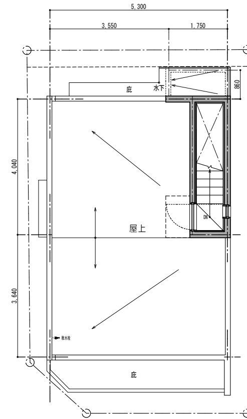
PH平面図
