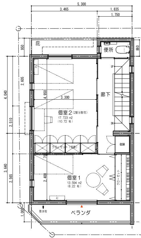
3階平面図
