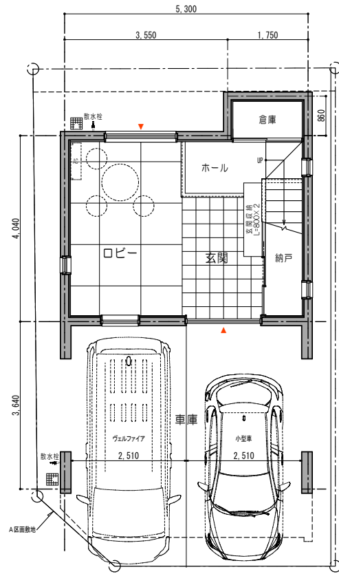
1階平面図
